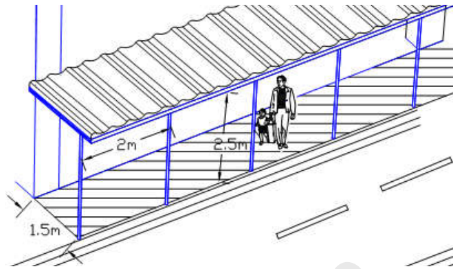
۸.۶. حصار حفاظتی موقت مطابق بند ۹-۵-۱۲
